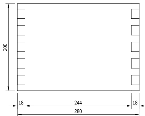
Pohled čelní
